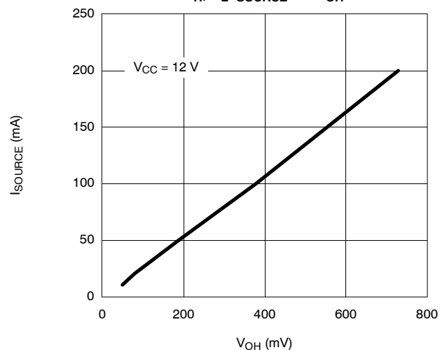
D_H, D_L I_{SOURCE} vs. V_{OH}
