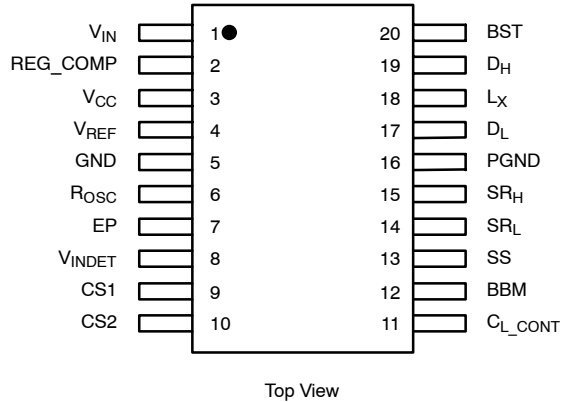
Si9122DQ (TSSOP-20)
