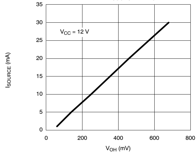
SRL, SRH I_{SOURCE} vs. V_{OH}
