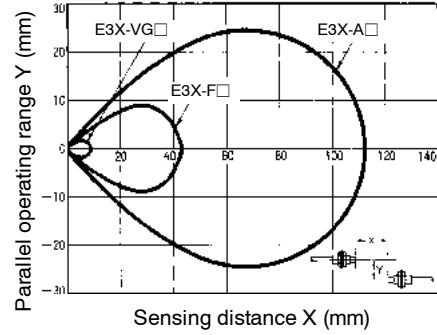
E32-TC200E with E3X-A, E3X-F and E3X-VG amplifiers
