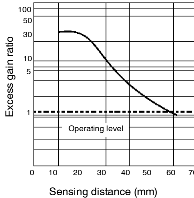
E32-D11 with E3X-A11 amplifier
