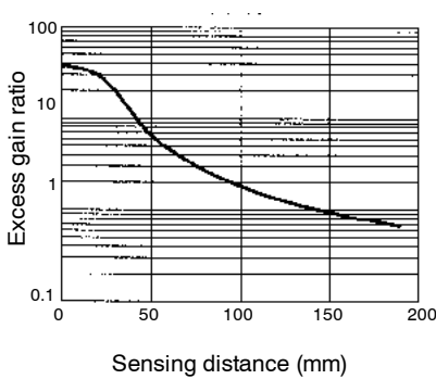
E32-JDBT1-3F with E3JU-X amplifier
