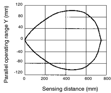
E32-UTBT1-6F with E3JU-X amplifier
