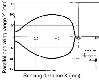
E32-T14L with E3X-NH amplifier
