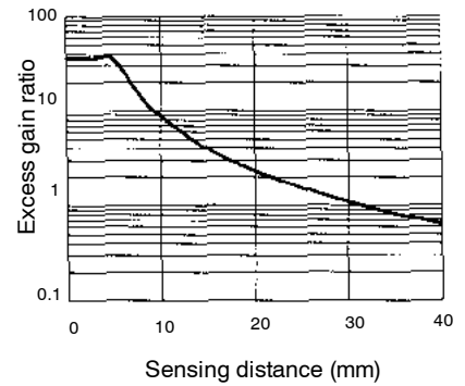
E32-D32 with E3JU-XR amplifier
