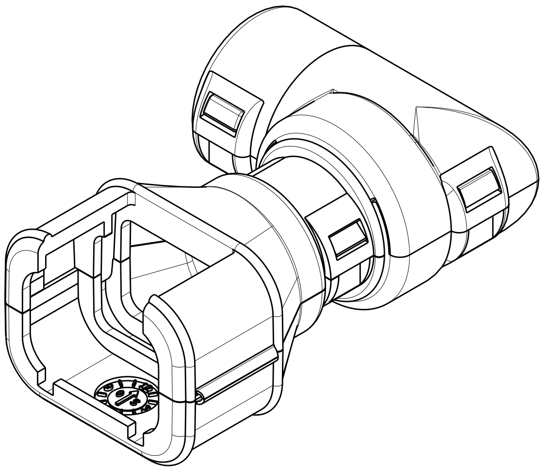
2035048-5 SCALE 3:1
