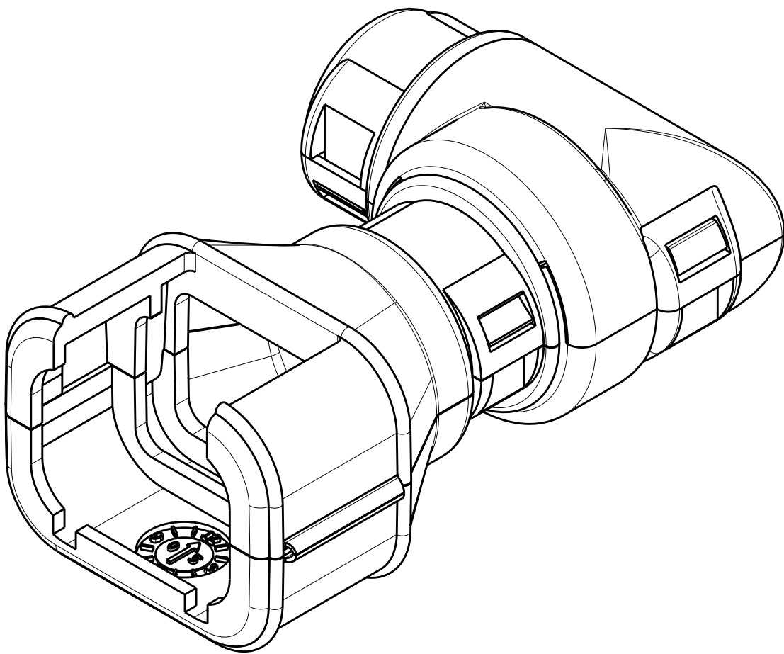
2035048-1 SCALE 3:1
