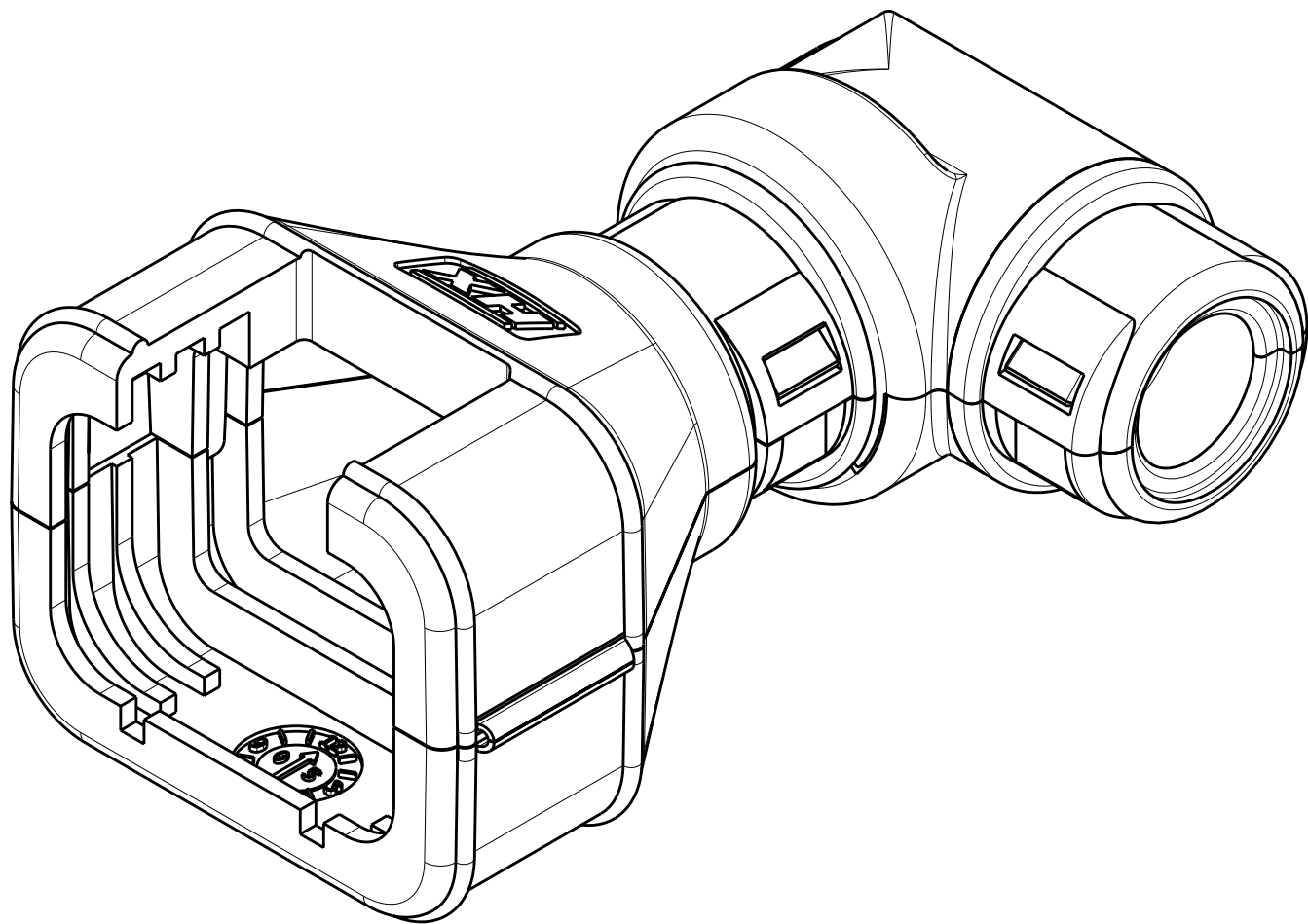
2035048-3 SCALE 3:1
