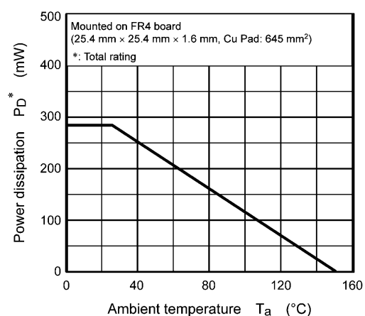
Fig. 7.14 P_D - T_a
