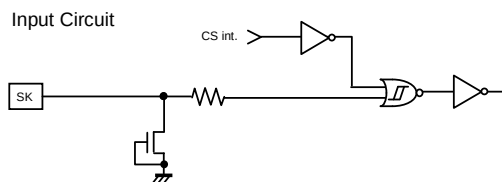
Figure 58. Input Circuit (SK)
