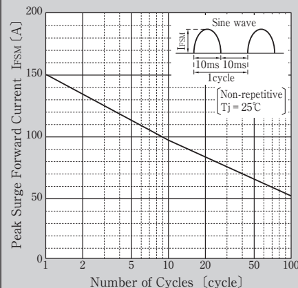
せん頭サージ順電流耐量
