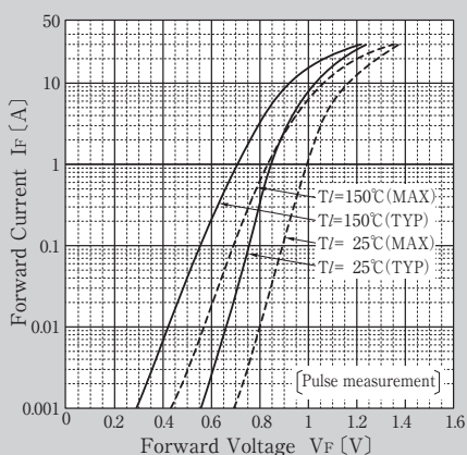
順方向特性
