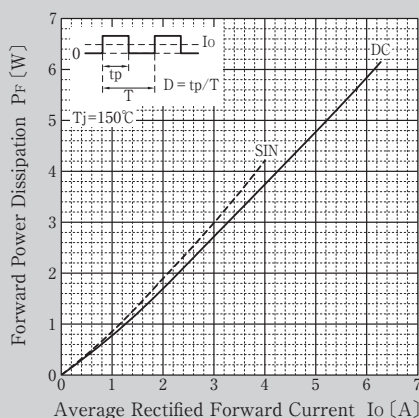
順電力損失曲線
