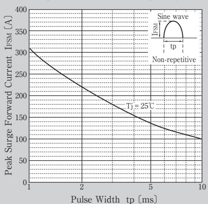
せん頭サージ順電流耐量
