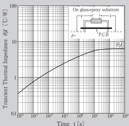
過渡熱抵抗
