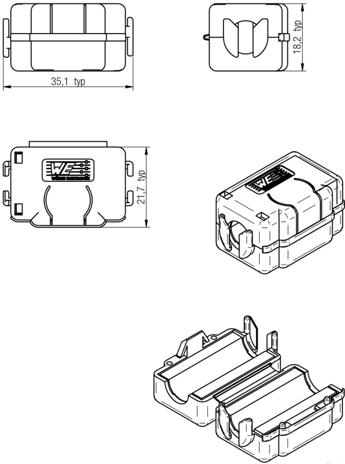
Scale - 1:1
