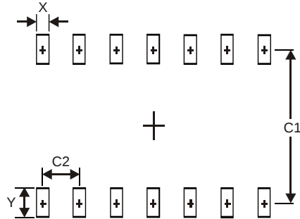
SO-14
