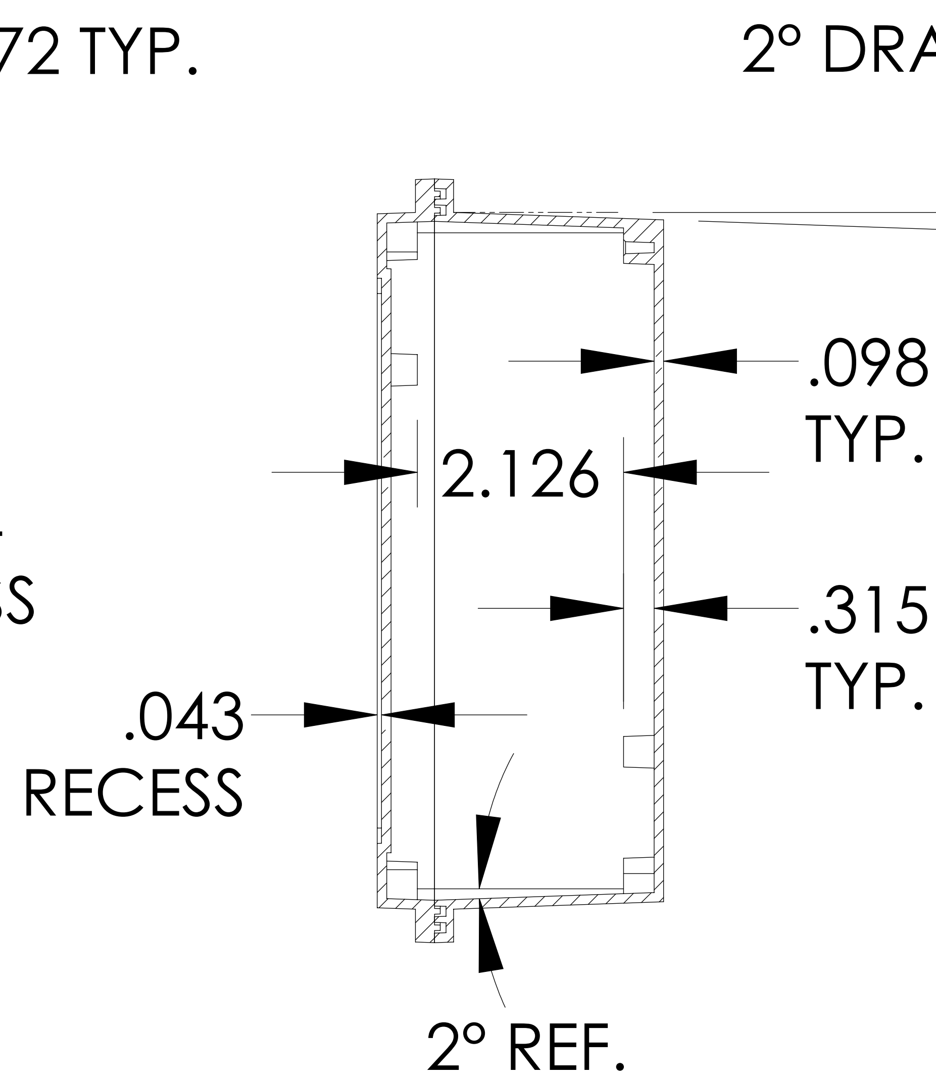
SECTION A-A
