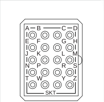
M81714/60-22-01 SHOWN
