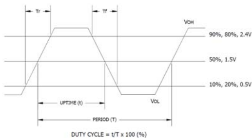
LVC MOS OUTPUT WAVEFORM
