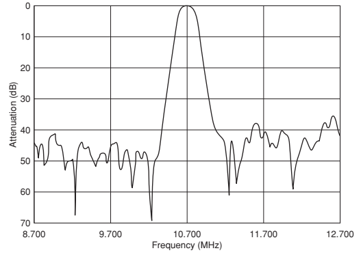
SFECF10M7GA00S0-R0/SFECF10M7GF00S0-R0
