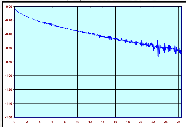
PN: CCSMA26.5-MM-086-5 INSERTION LOSS (S21)
