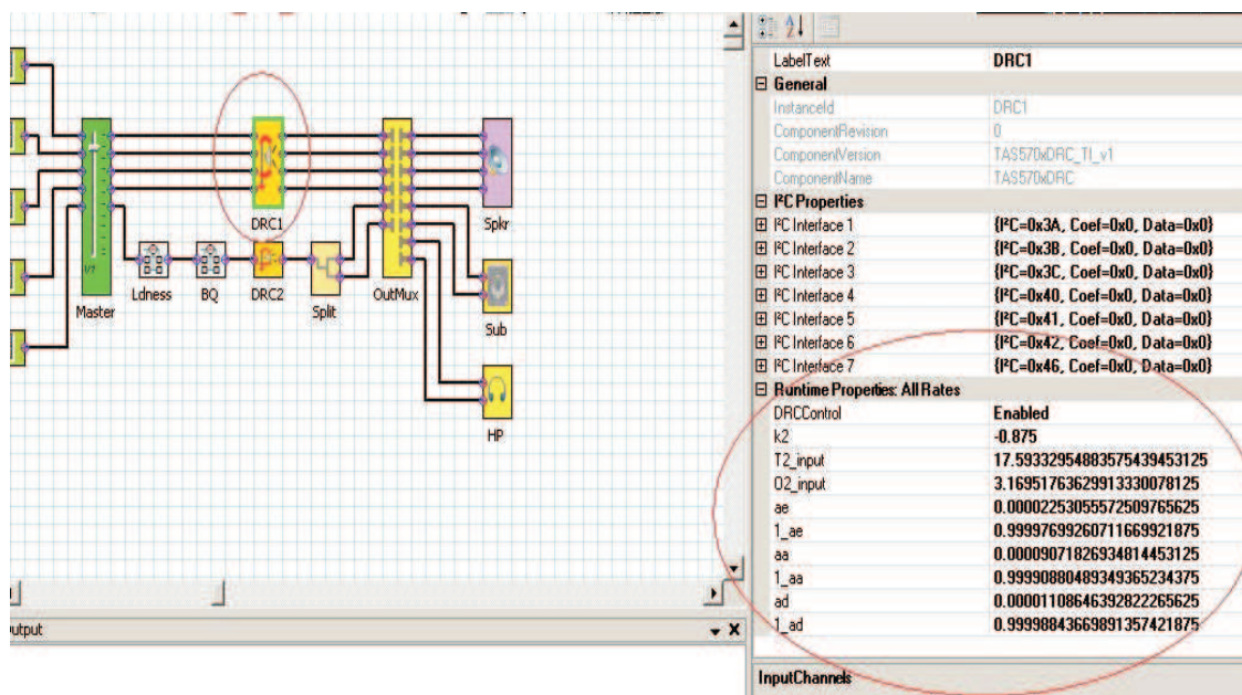
Figure 16. DRC Parameters
