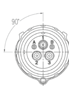
STRAIGHT PLUG STECKER, GERADE CONNECTEUR DROIT
