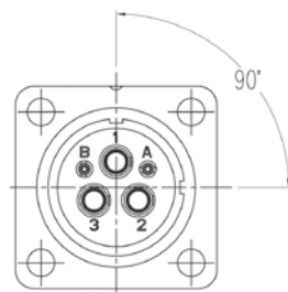
RECEPTACLE STECKDOSE EMBASE
