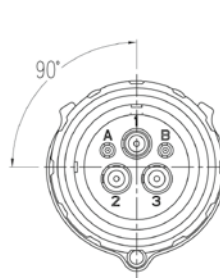
STRAIGHT PLUG STECKER, GERADE CONNECTEUR DROIT
