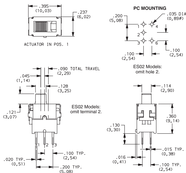
ES01MCBE SPDT
