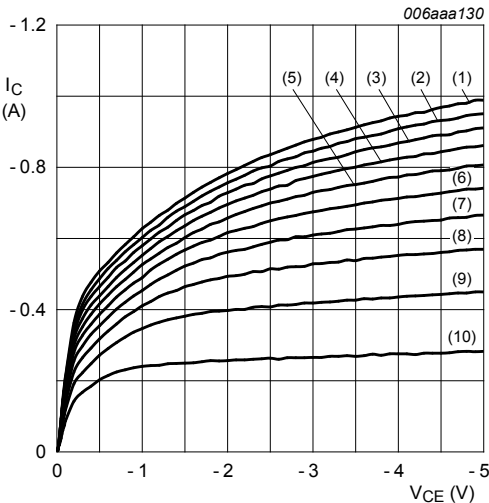
T_{amb} = 25\text{ °C} (1) I_B = -12.0\text{ mA} (2) I_B = -10.8\text{ mA} (3) I_B = -9.6\text{ mA} (4) I_B = -8.4\text{ mA} (5) I_B = -7.2\text{ mA} (6) I_B = -6.0\text{ mA} (7) I_B = -4.8\text{ mA} (8) I_B = -3.6\text{ mA} (9) I_B = -2.4\text{ mA} (10) I_B = -1.2\text{ mA}
