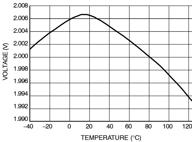
Figure 20. V ref_EN
