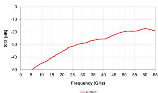
S12
