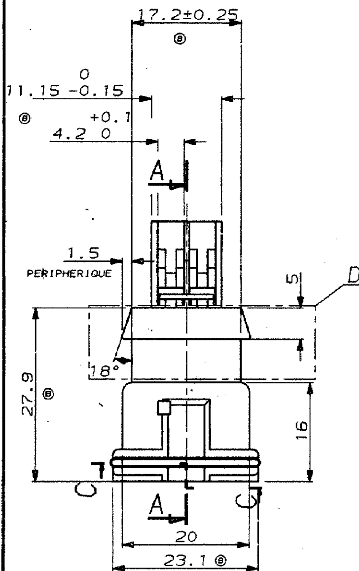
DETAIL D: PARTIE SUPERIEURE PORTE-MODULE
