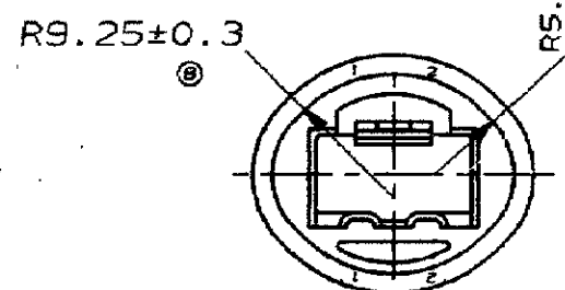
DETAIL D: PARTIE SUPERIEURE PORTE-MODULE
