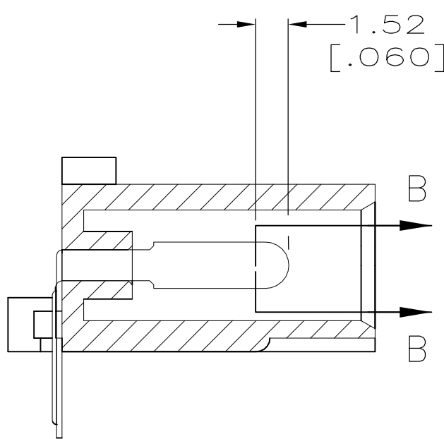
SECTION A-A
