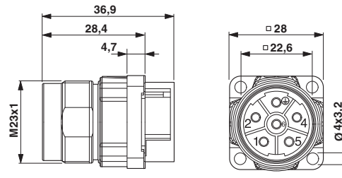
Installation dimensions SF-...P1N8AWK00
