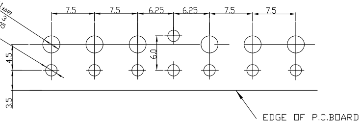
LAY-OUT P.C.B.- HOLE
