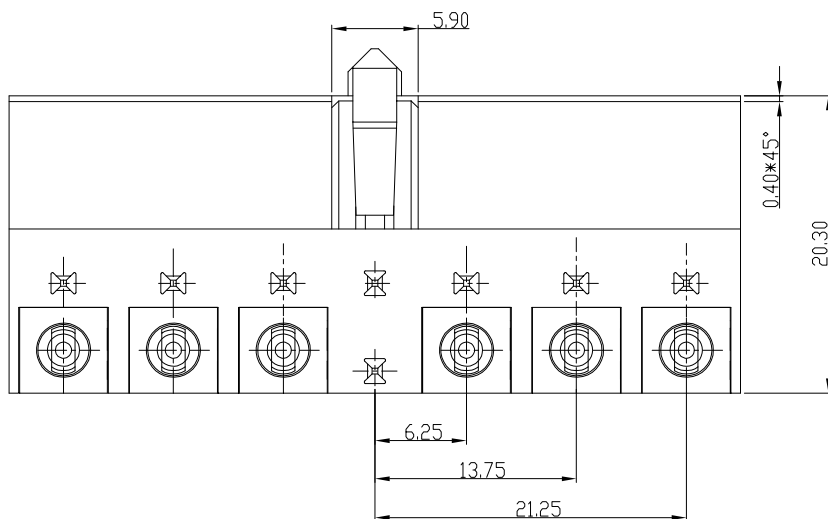
LAY-OUT P.C.B.- HOLE
