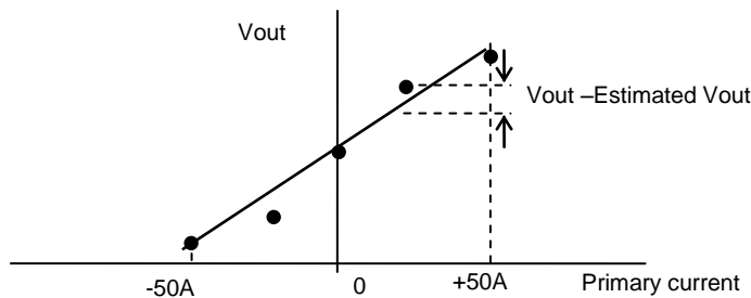
Fig.8-1 Non linearity
