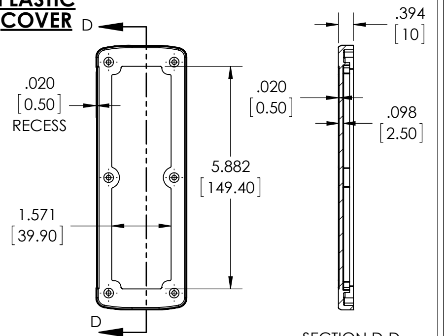
SECTION D-D
