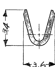
A-A 断面
