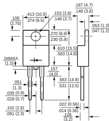
TO-220A
