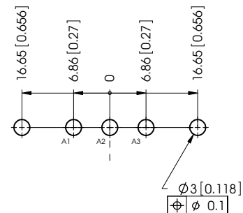
FM3W3 / F3W3...C
