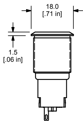
FLAT ACTUATOR
