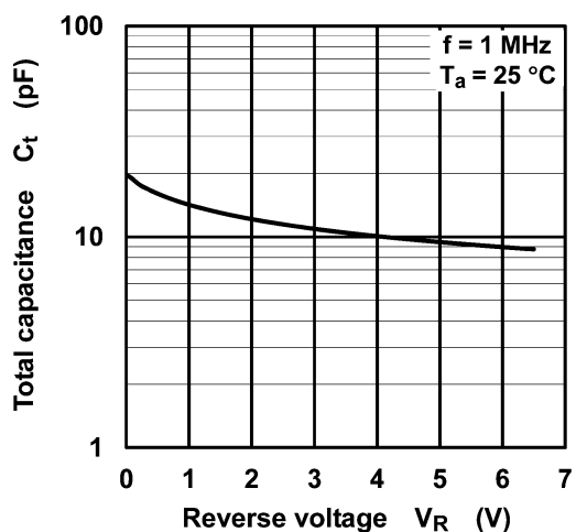
Fig. 8.3 C_t - V_R
