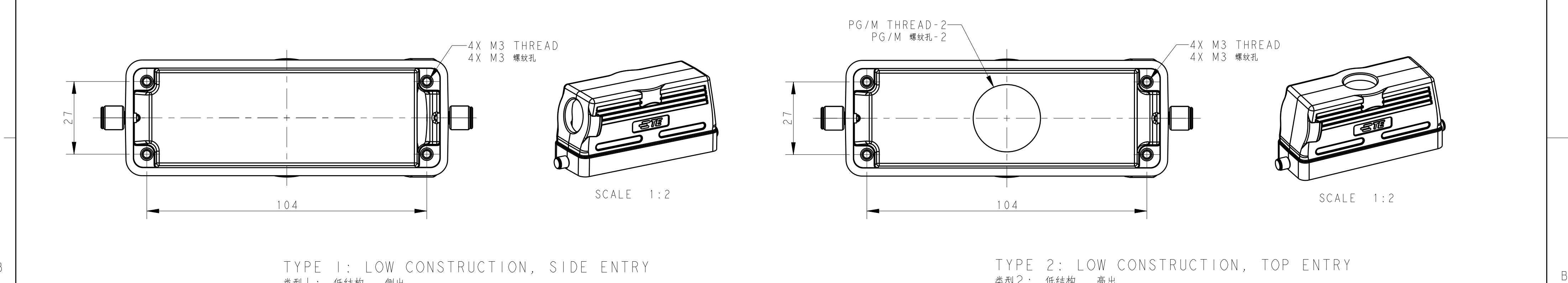
TYPE 1: LOW CONSTRUCTION, SIDE ENTRY 类型1: 低结构, 侧出 TYPE 2: LOW CONSTRUCTION, TOP ENTRY 类型2: 低结构, 高出
