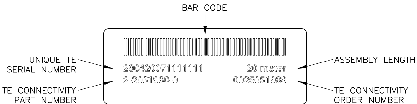
3 LABEL DETAIL:
