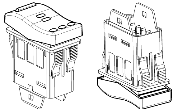
3251 Serie: Grundschafter 3250 mit Kappe 3251 series: basic switch 3250 with cap
