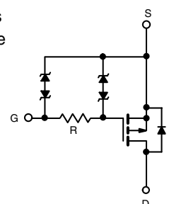
P-Channel MOSFET
