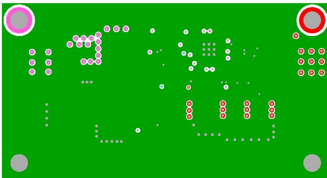
FIGURE 26. LAYER 3
