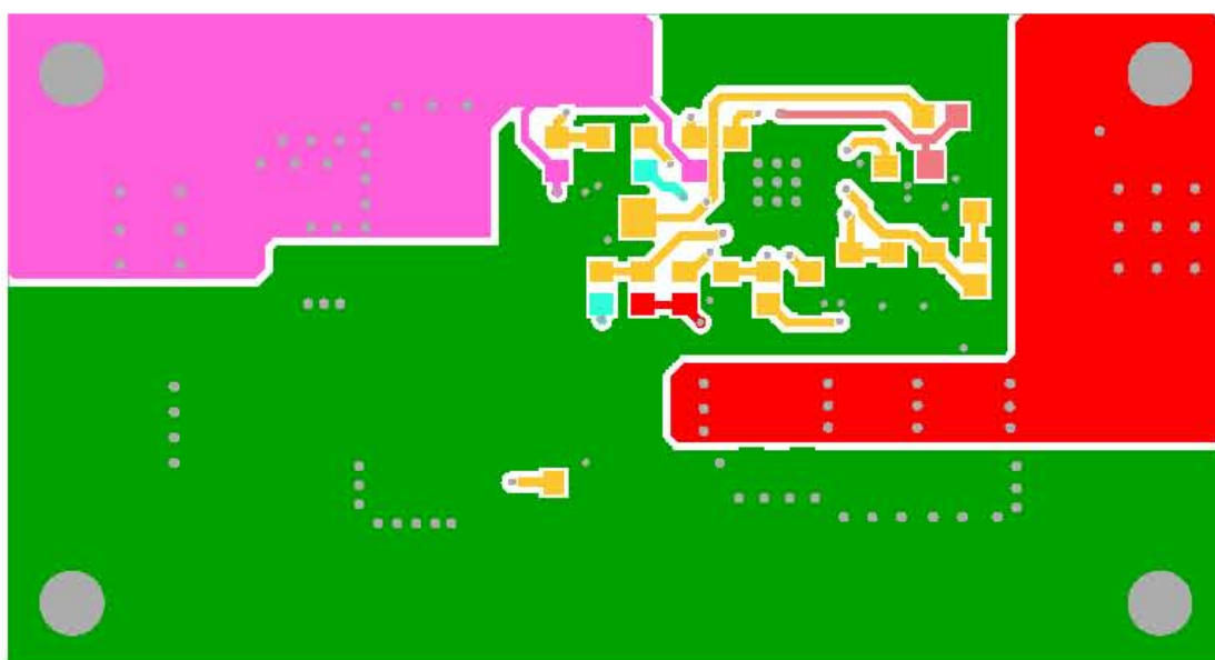
FIGURE 27. BOTTOM LAYER
