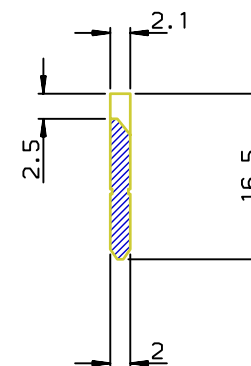
COUPE AA
