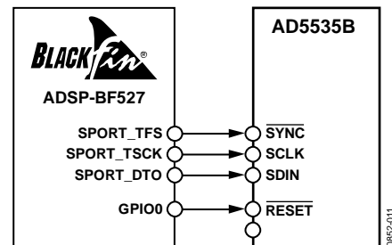
Figure 16. AD5535B -to-ADSP-BF527 Interface
