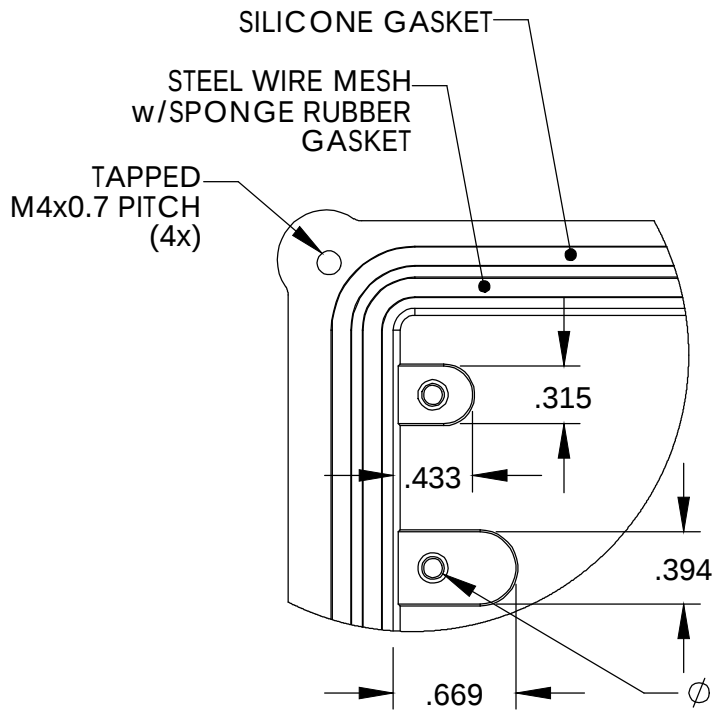
SCALE 4 : 1
