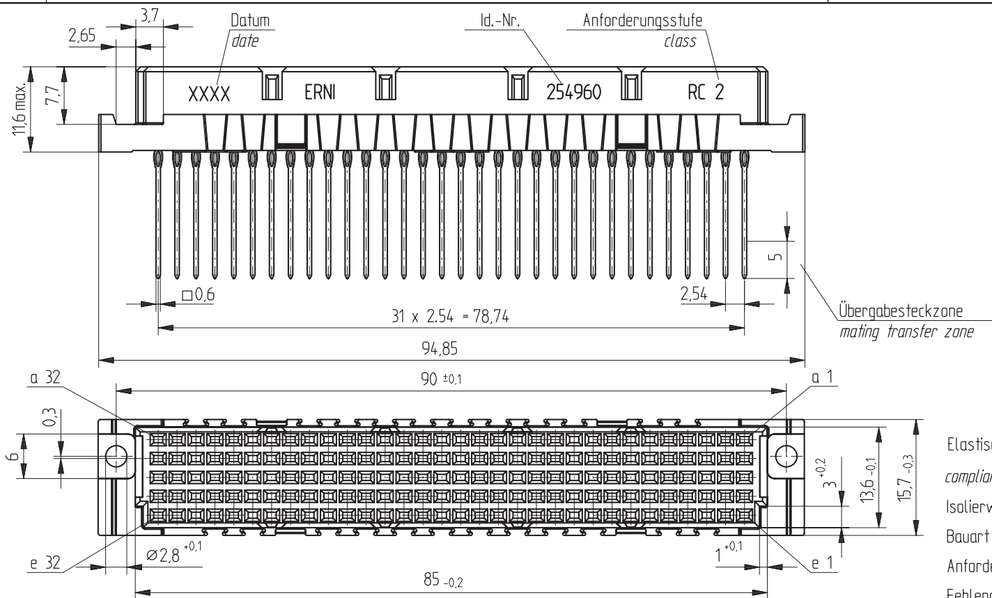
Bestückungsplan / contact layout
