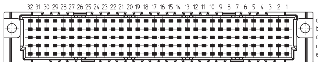
Leiterplatten-Lochbild / PCB drillhole pattern
