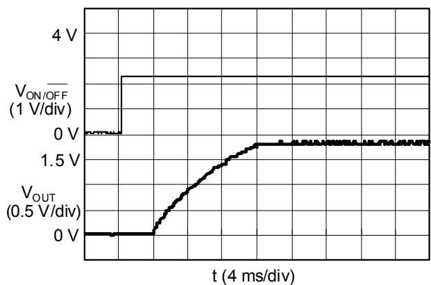
(5) S-8540A18FN ( V_{\text{IN}} : 4.95 \text{ V} )
