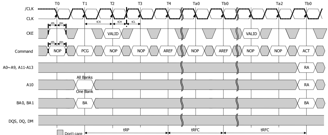
Figure33 : Auto refresh
