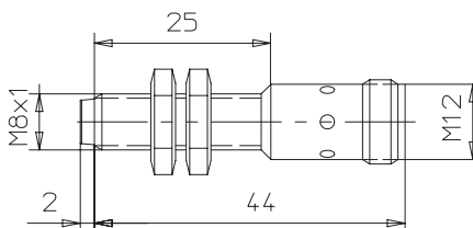
E2EL-X2M□-M1
