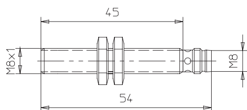
E2EL-X1R5□-M3L, E2EL-X2□DM3S
