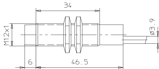
E2EL-X4M□-L 2M
