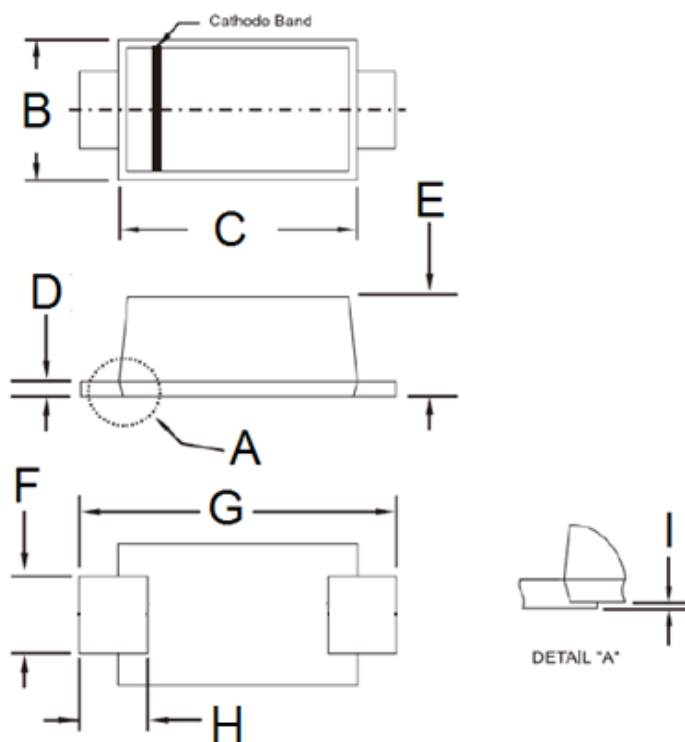
SOD-123W
