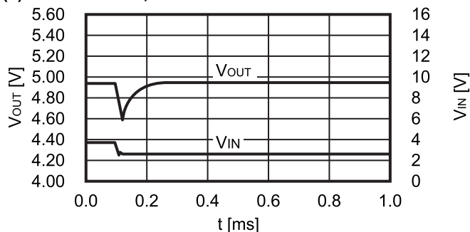
(2) f_{osc} = 1.2\text{ MHz} , V_{IN} = 3.8\text{ V} \rightarrow 2.8\text{ V} S-8365AABBA
