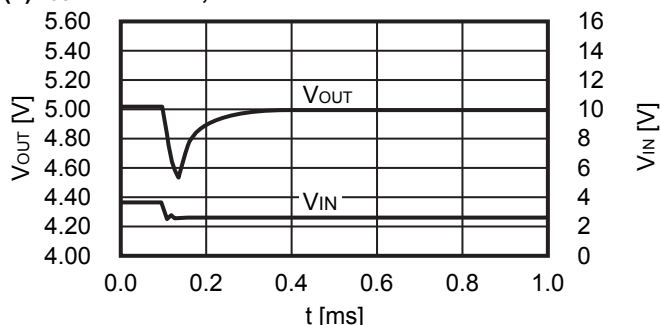
(4) f_{osc} = 600\text{ kHz} , V_{IN} = 3.8\text{ V} \rightarrow 2.8\text{ V} S-8365ABBBA
