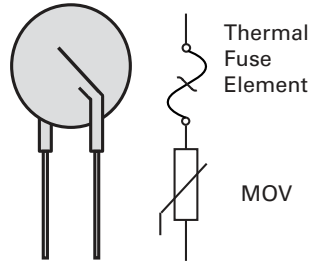
TMOV® Varistor
