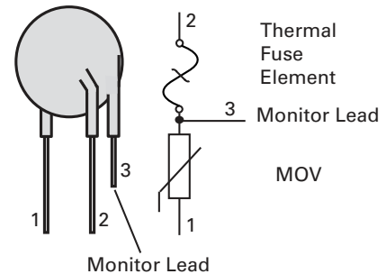
iTMOV® Varistor
